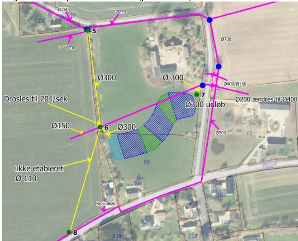
Bilag 2: Kort over de nye rør der leder vand til og fra minivådområdet
